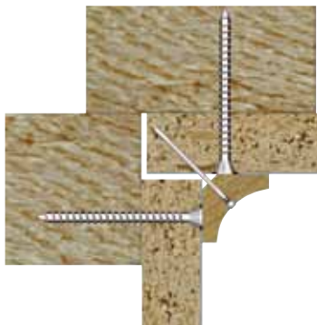
Fig. 5 Innvendig hulkillist
