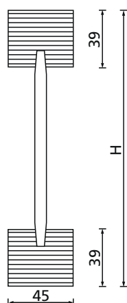
Hunton I-bjelken SJ45
