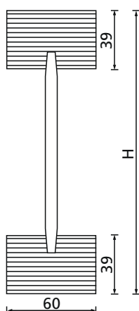
Hunton I-bjelken SJ60
