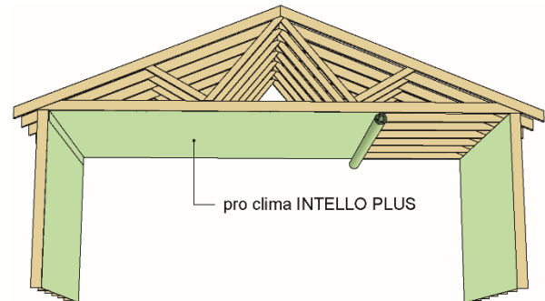
Fig. 1 pro clima INTELLO PLUS montert i yttervegg og mot kaldt loftstom
