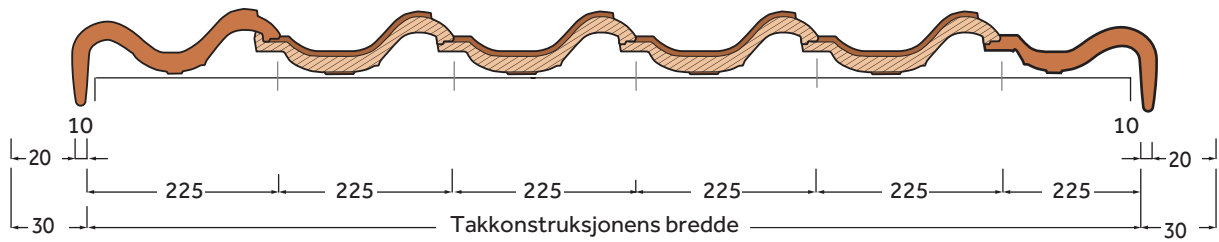
Figur 14: Hollander V med gavlstein
