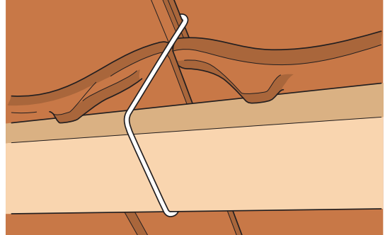
Figur 6: Feste med M-Clip
