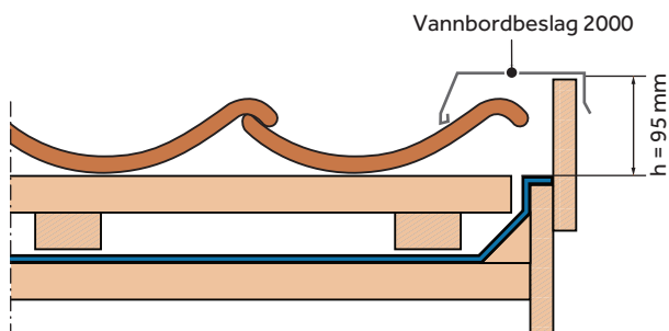
Figur 16: Konstruksjonsbredde uten bruk av gavlstein for Hollander V tegltakstein
