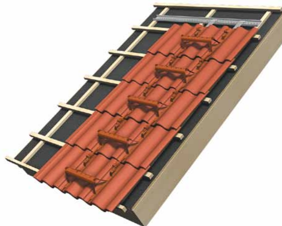
Bilde 13. Stigetrinn
