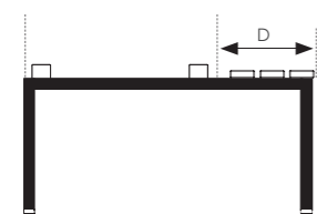
Helsveiset sittebenk med justerskruer Sitteflate i lakkert furu eller grå laminat. Høyde: 400 mm. D: 300 mm Farge RAL 7021.
