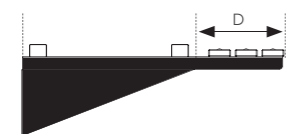
Sittebenk for veggmontering D: 284 mm Sitteflate i lakkert furu eller grå laminat.
