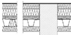
Snitt av korrugert stålplatetak
