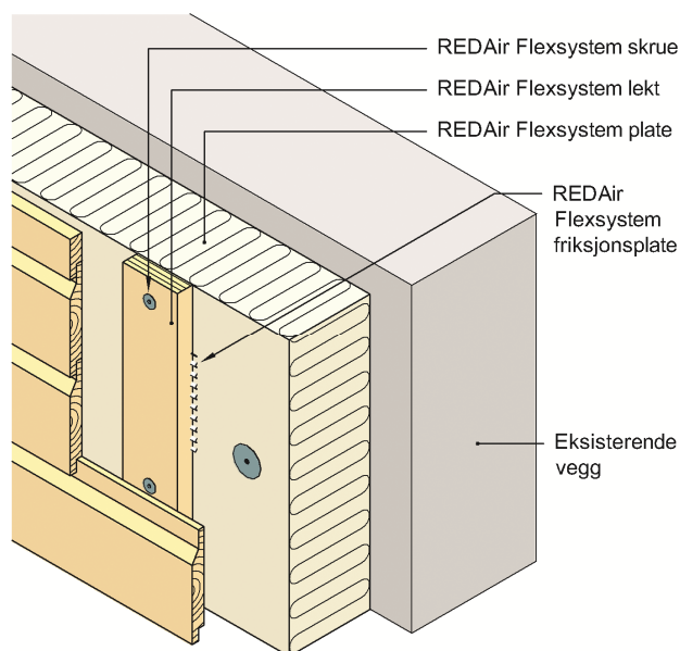
Fig. 1 Rockwool REDAir Flexsystem
