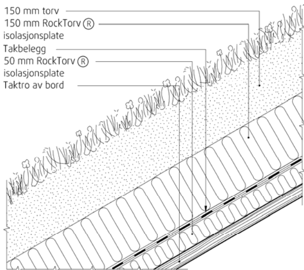
Fig. 5 Eksempel på Rockwool Torvtak med tilleggisolasjon under takbelegget.
