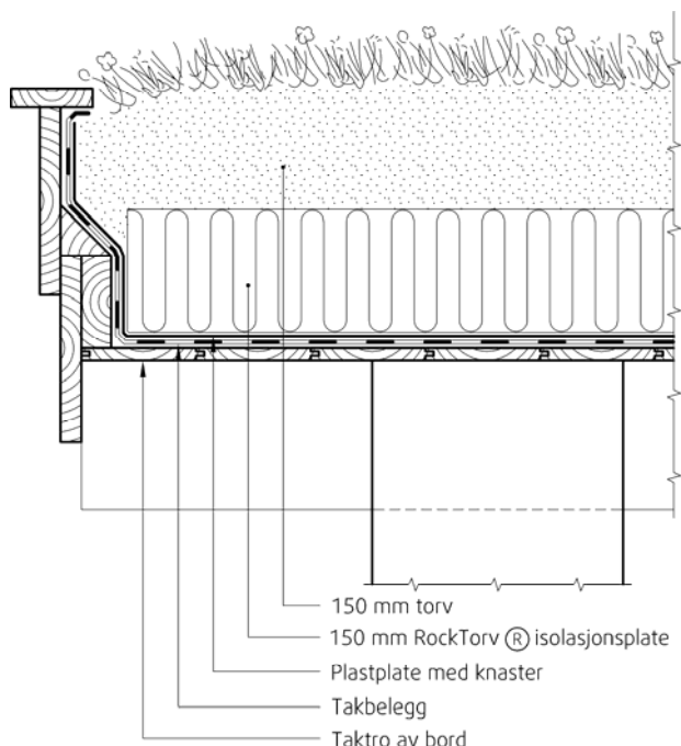
Fig. 3 Eksempel på takutstikk på gavli med Rockwool Torvtak. Med stor tykkelse på varmeisolasjonen kan det være behov for bruk av flere vindskier.
