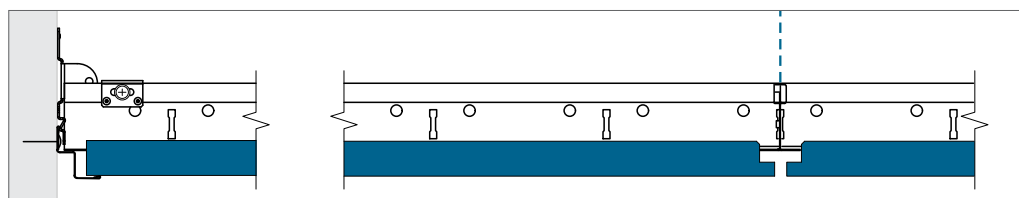
Kantdetalj ved tværrøfil
