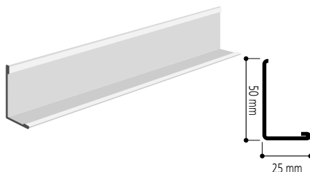
Kantprofil 1421 for SY-XL
