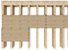
Montering af gulvplader på træstrøer
