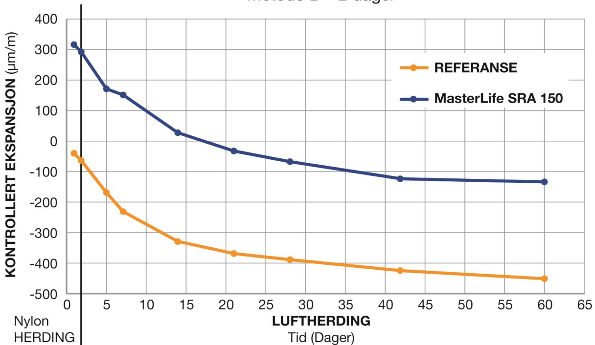
Fig. 1: Kontrollert ekspansjon etter UNI8148 med MasterLife SRA 150
