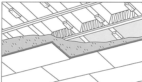
Nedlekting for himlingspalter, med understøtting.
