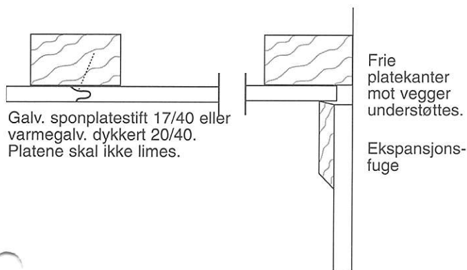
Platene montert direkte på bjelkene.
