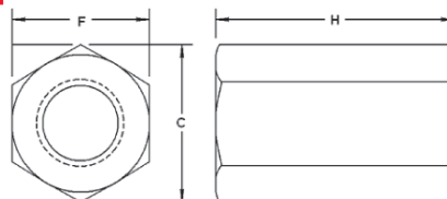
Skjøtemutter DIN 6334
