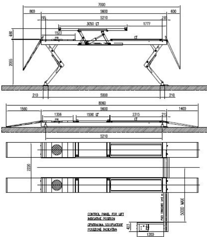
Målskisse KAR55 5600mm m/gjennomkjøring
