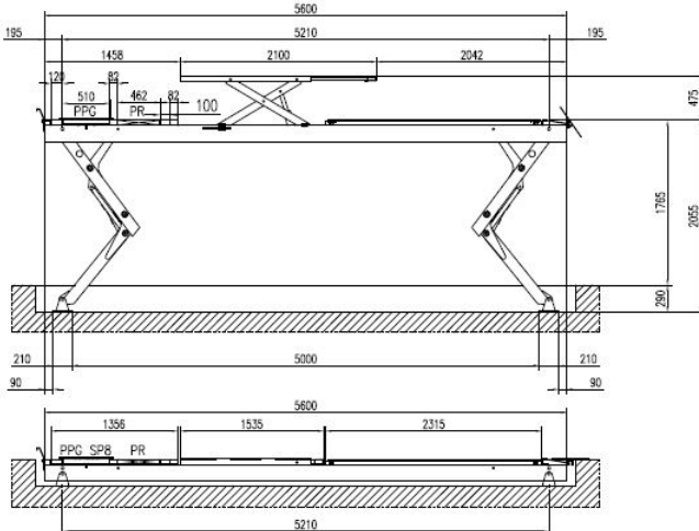
Målskisse KAR55 5600 I Gulv
