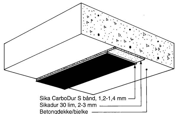
Fig. 1 Snitt av armert betongkonstruksjon forsterket med utenpåliggende Sika CarboDur S bånd på strekksiden
