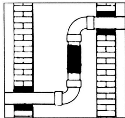
Gjennomføringer o.l. i murverk
