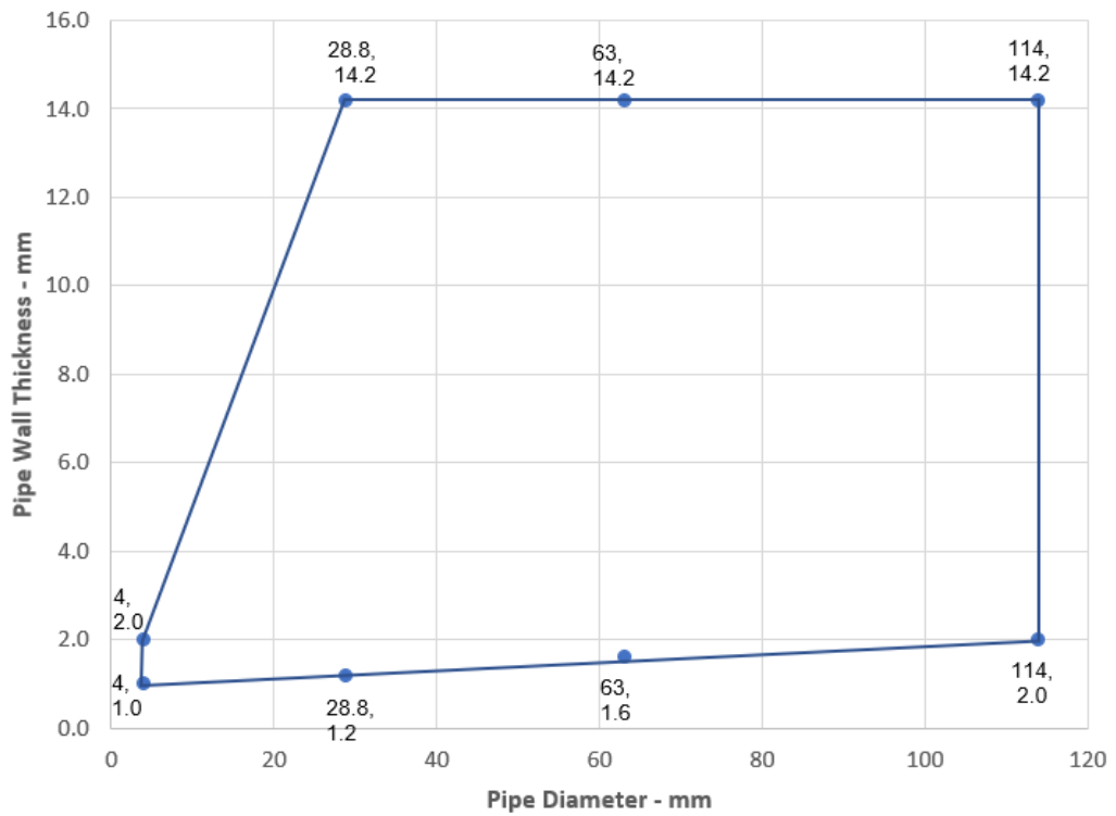
Steel Pipes - E 90 C/C, EI 45 C/C
