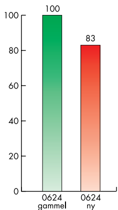
Sammenlikning av dreiemoment i % Bor Ø6mm boreddybde 18mm
