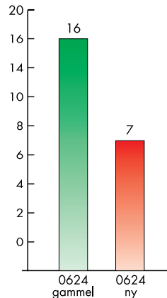
Sammenlikning av boretid Bor Ø 6mm boreddybde 10mm
