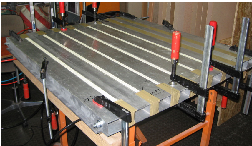
Abbildung 1 Geschäumte Fugen in Prüfvorrichtung für Längsfugen nach DIN 18542, aufgespannt auf eine luftdichte Edelstahlwanne als Prüfkammer
