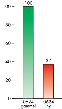
Sammenlikning av boretid Bor Ø 6mm boreddybde 10mm
