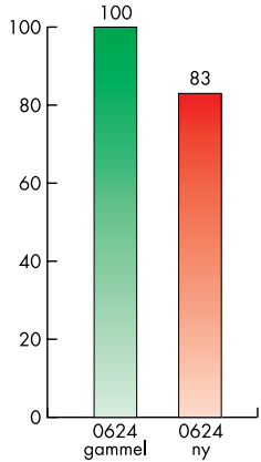
Sammenlikning av dreiemoment i % Bor Ø6mm boreddybde 18mm
