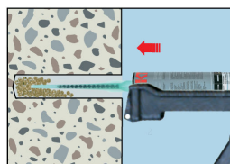
Mørtel injiseres
