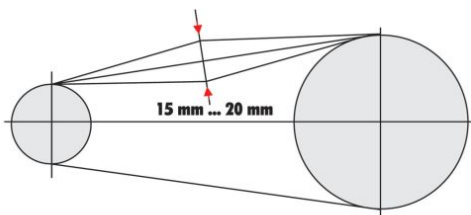
treibendes Rad
