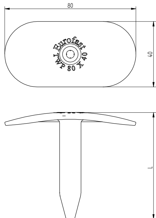
Eurofast TWP-8040
