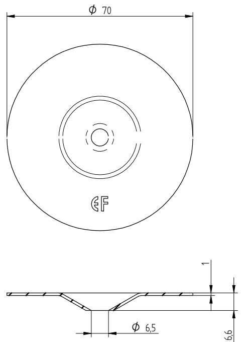
Eurofast DVP-EF-7010D
