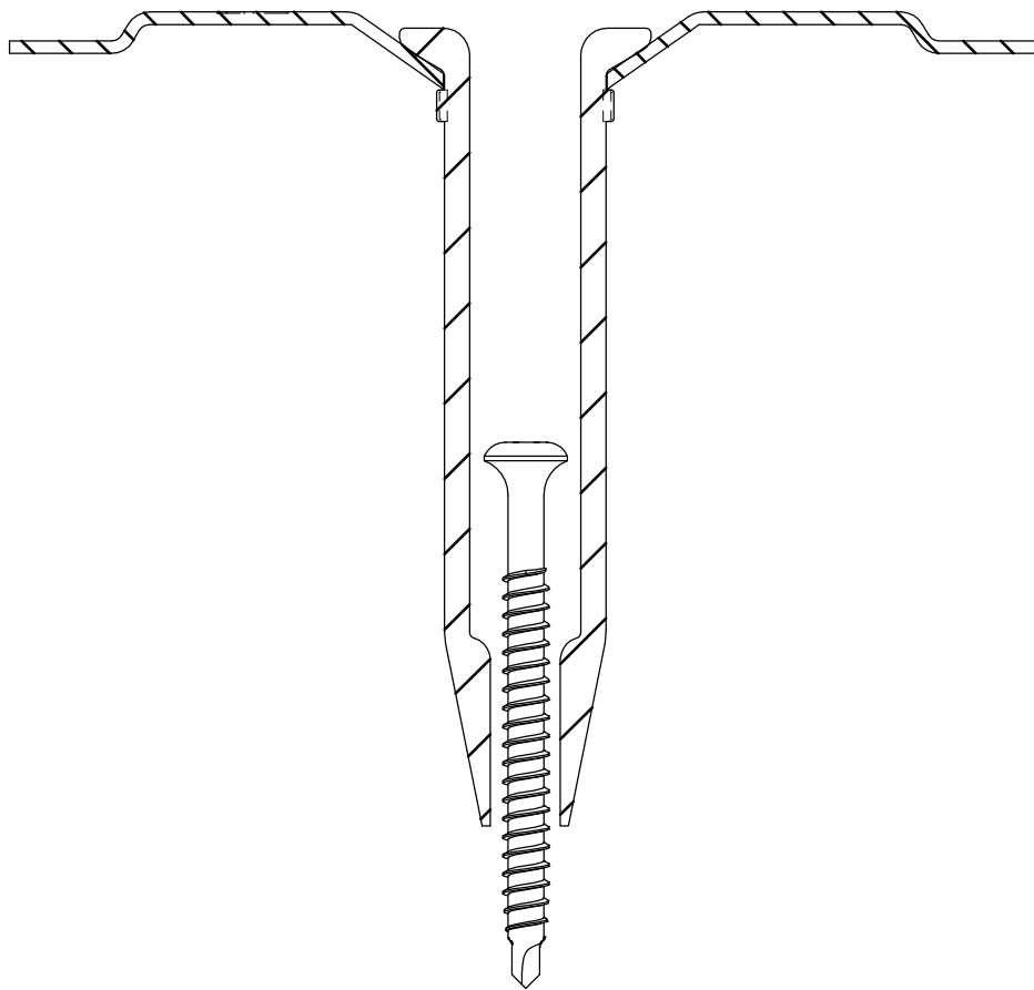
Eurofast EDS-SRB 4,8 x L
