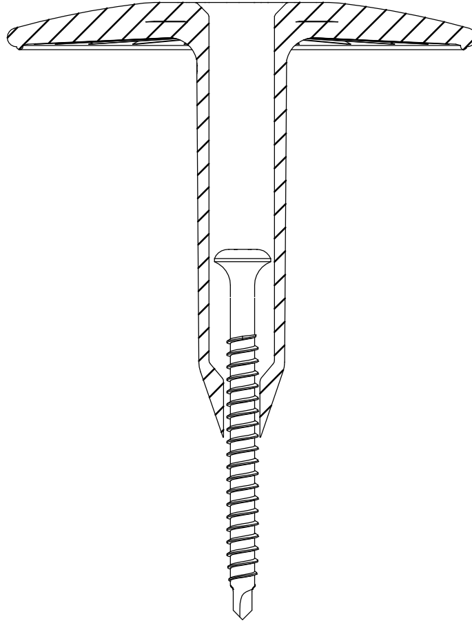
Eurofast TLK-75
