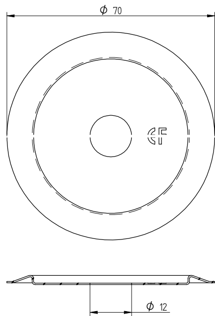
Eurofast DVP-ISPC-70N
