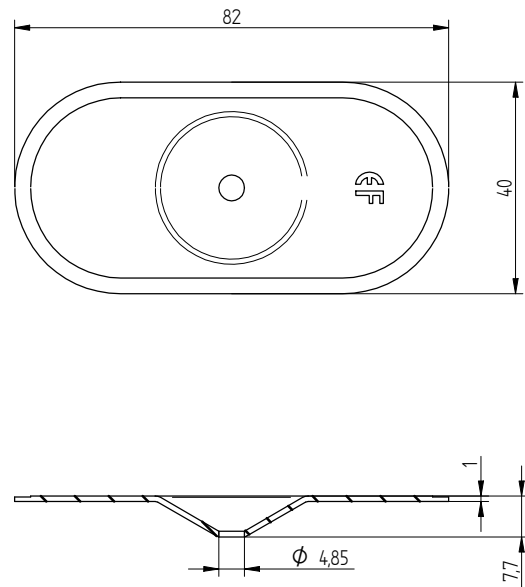
Eurofast DVP-EF-8240D
