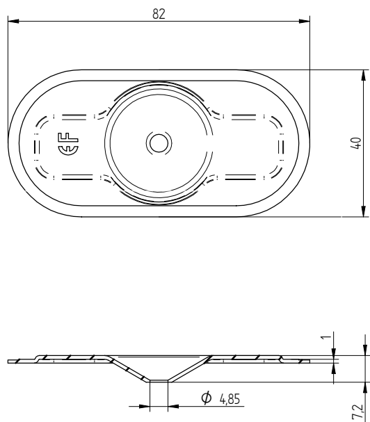
Eurofast DVPEFZK8240D
