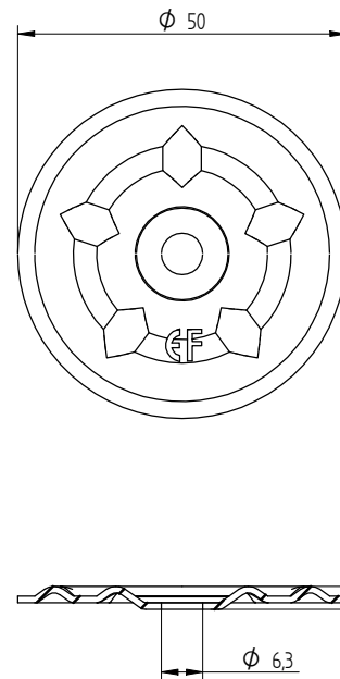
Eurofast DVP-EF-5010N
