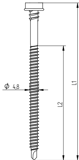
Eurofast EDS-BZTR 4,8 x L
