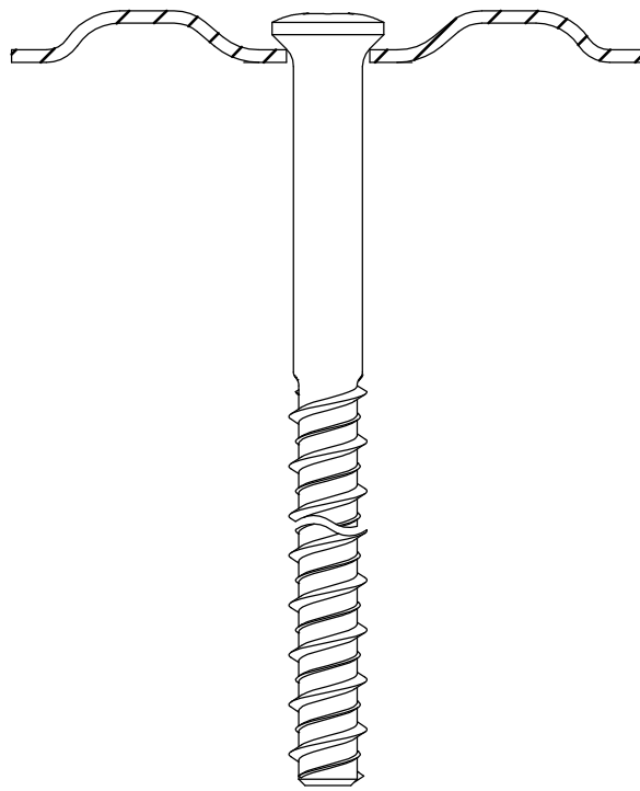
Eurofast DVP-EF-51N
