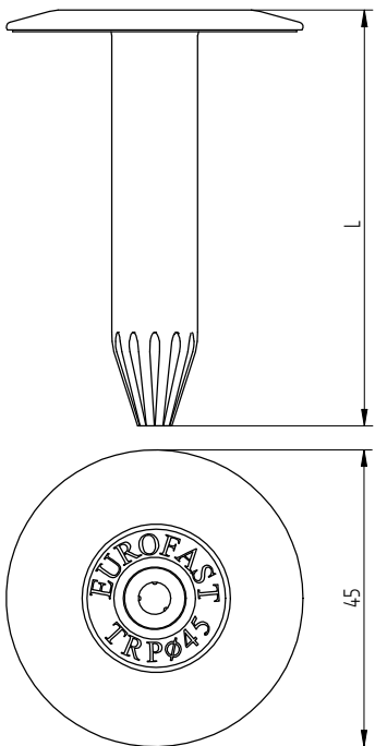
Eurofast TRP-45
