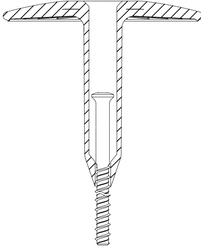
Eurofast TLK-75
