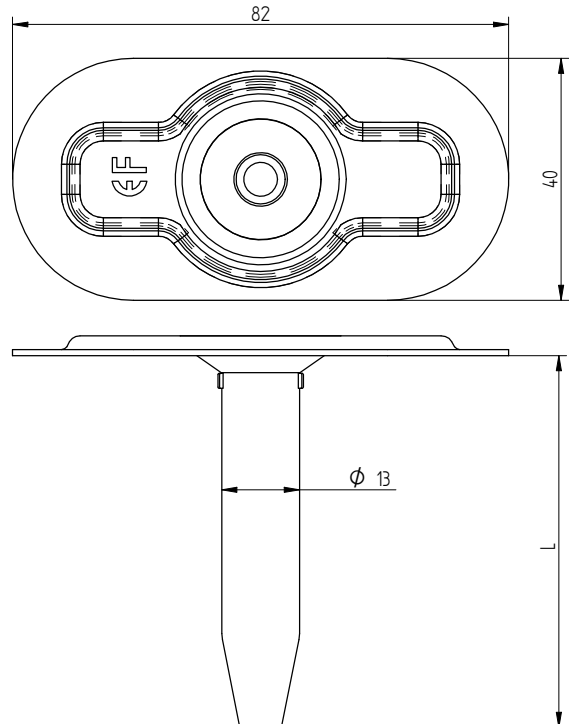
Eurofast KMT-15 Eurofast DVPKMT-8240D
