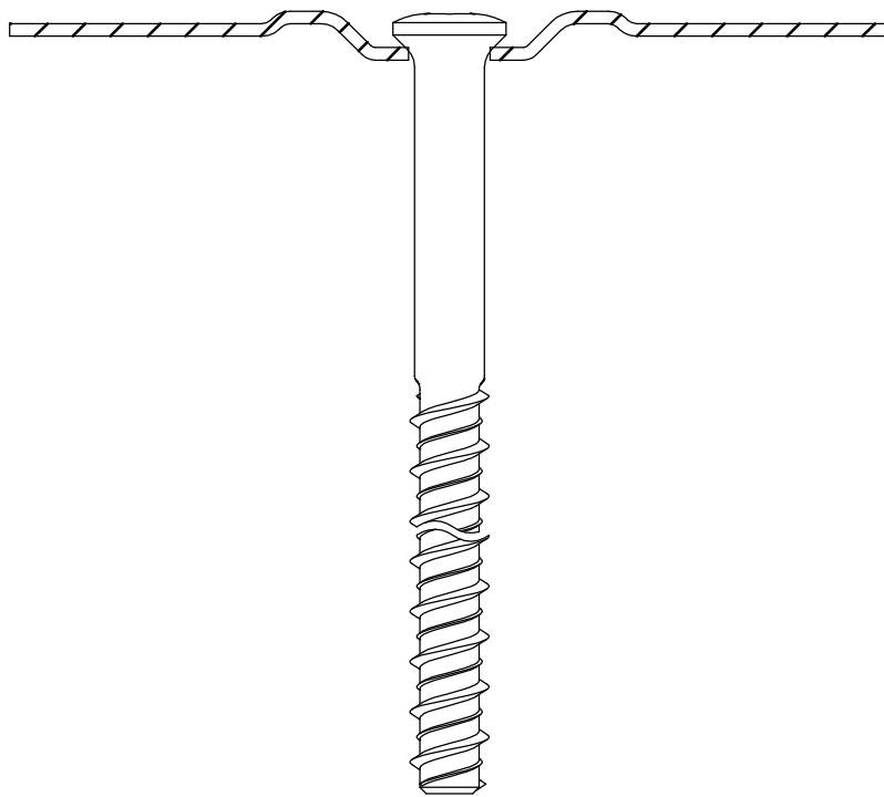
Eurofast EFR 6,3 x L
