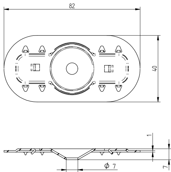
Eurofast DVP-DFB8240D
