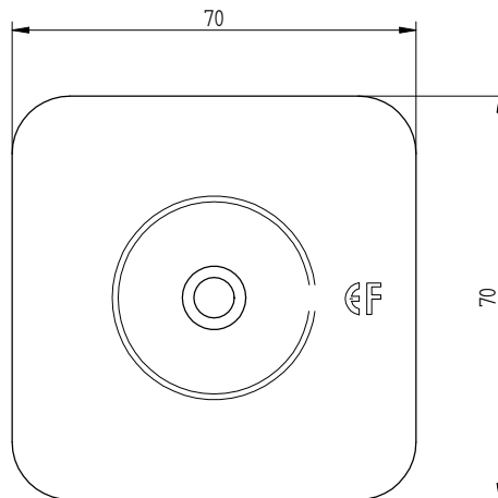
Eurofast DVP-DF-7070D
