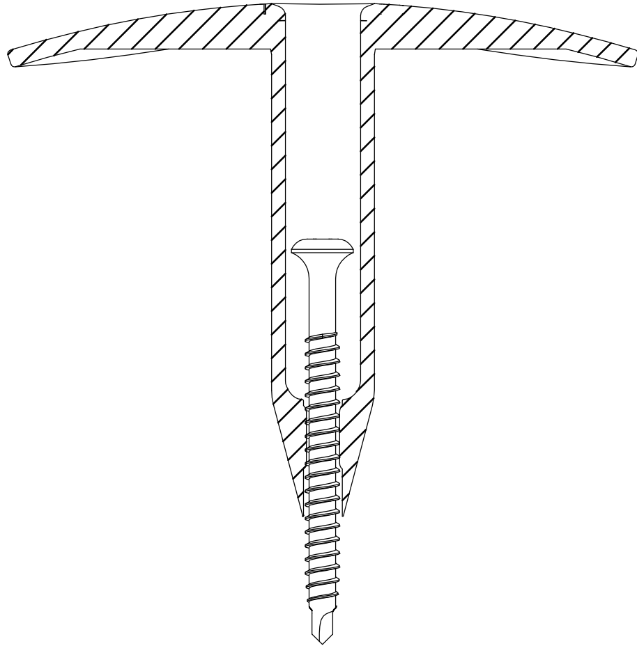
Eurofast TWP-8040
