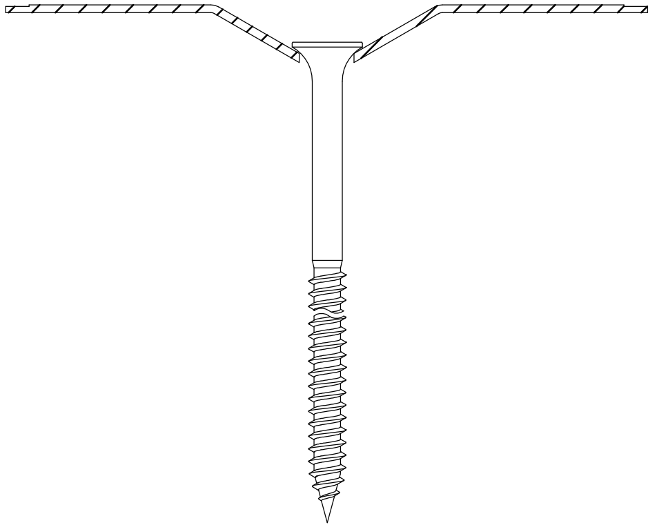
Eurofast EDS-S 4,8 x L
