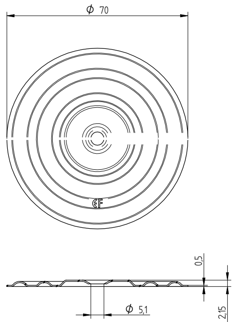
Eurofast DVP-EF-7005N
