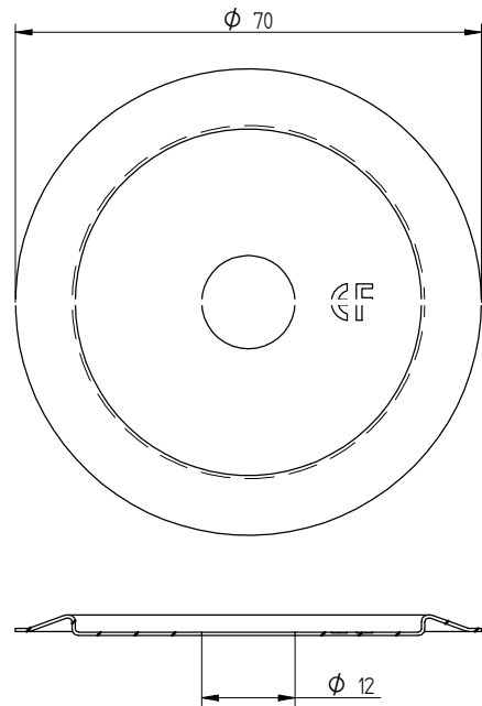
Eurofast DVP-ISPC-70N
