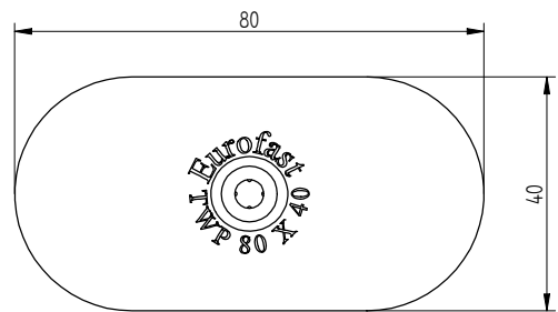
Eurofast TWP-8040
