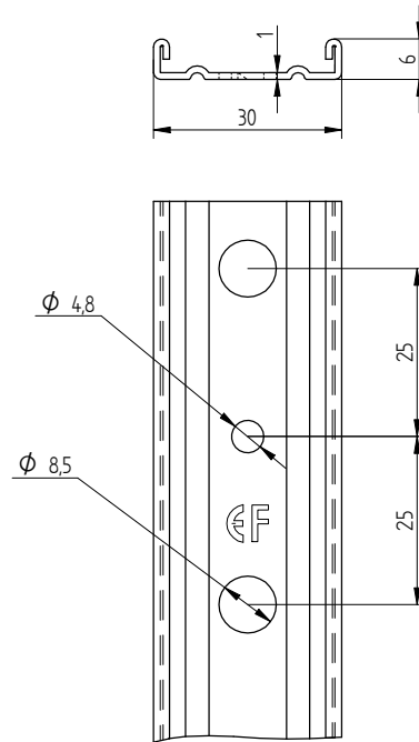
Eurofast EDF-BAR-F
