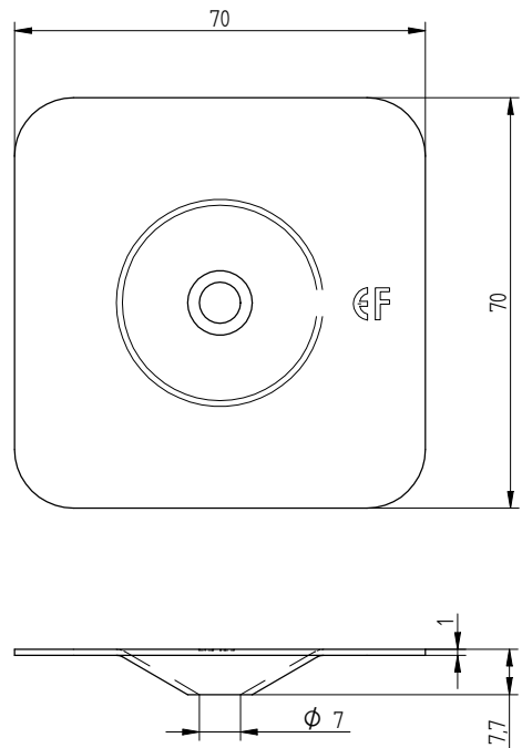
Eurofast DVP-DF-7070D
