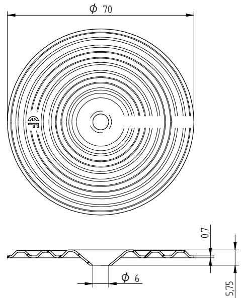
Eurofast DVP-EF-7007D
