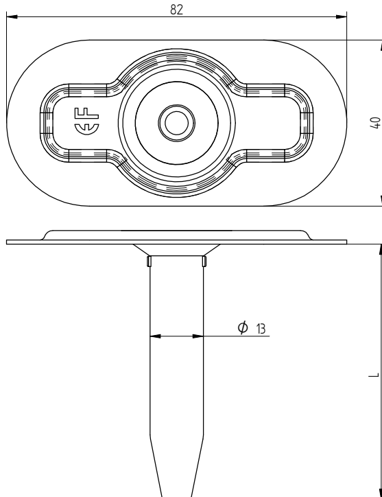
Eurofast KMT-15 Eurofast DVPKMT-8240D
