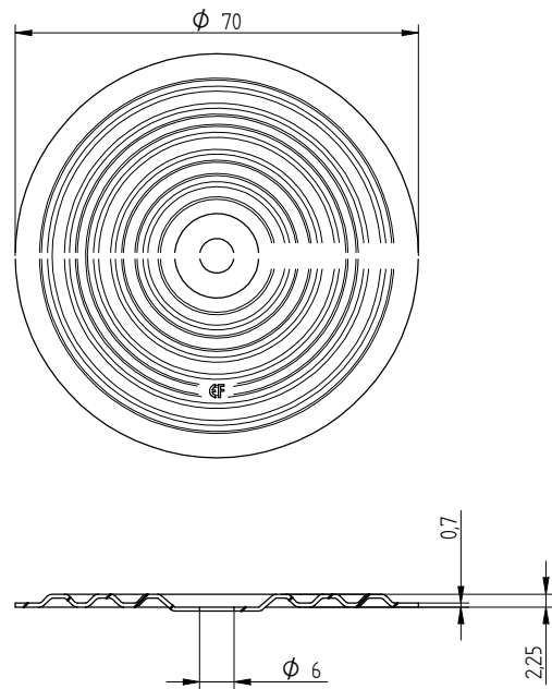
Eurofast DVP-EF-7007N
