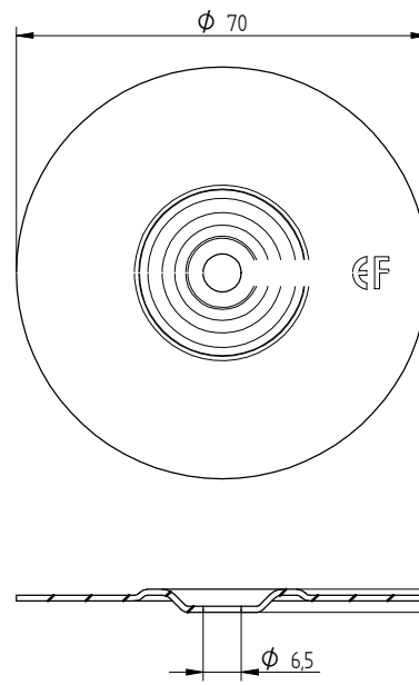
Eurofast DVP-EF-7010N
