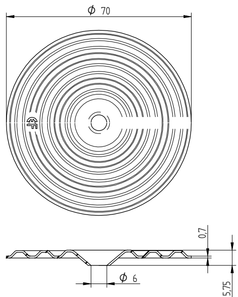
Eurofast DVP-EF-7007D
