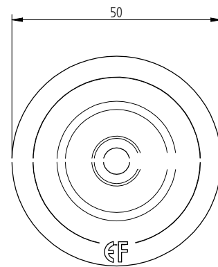
Eurofast DVP-EF-5010D
