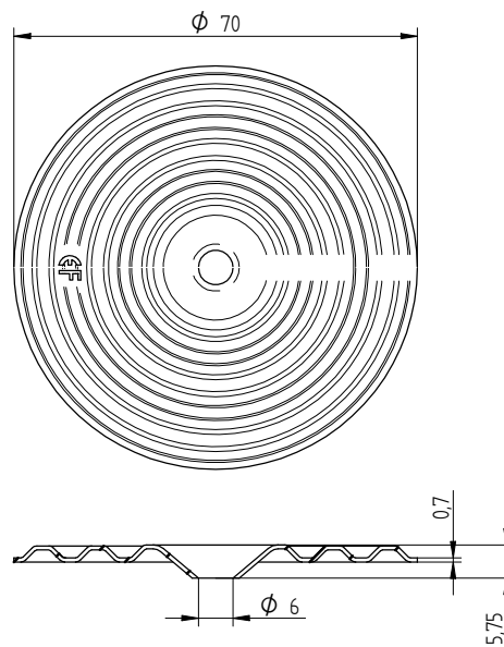
Eurofast DVP-EF-7007D
