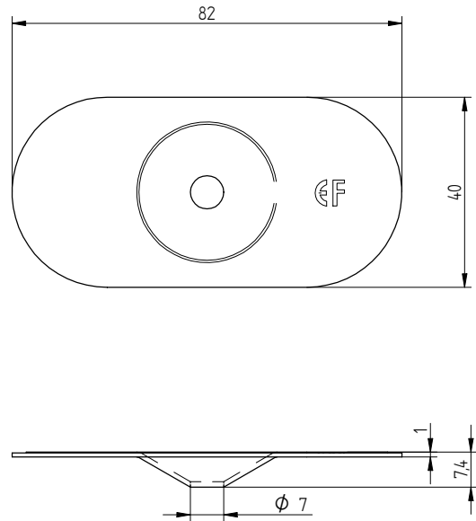
Eurofast DVP-DF-8240D
