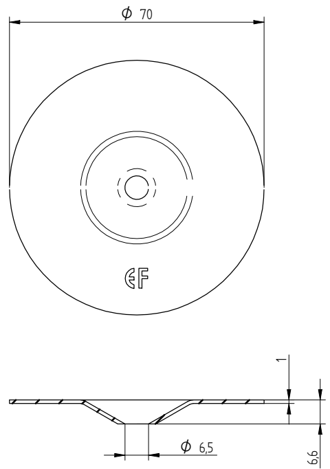
Eurofast DVP-EF-7010D
