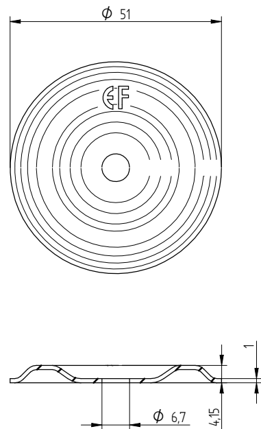
Eurofast DVP-EF-51N
