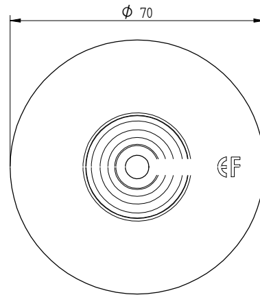
Eurofast DVP-EF-7010N
