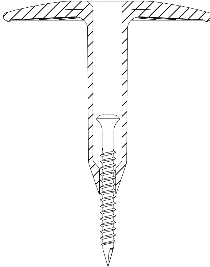
Eurofast TLK-75
