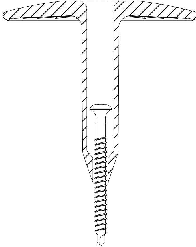
Eurofast TLK-75
