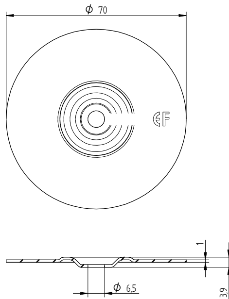
Eurofast DVP-EF-7010N
