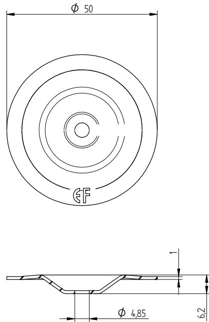
Eurofast DVP-EF-5010DFR
