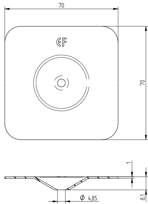
Eurofast DVP-EF-7070D
