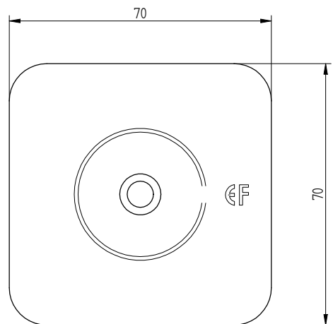
Eurofast DVP-DF-7070D
