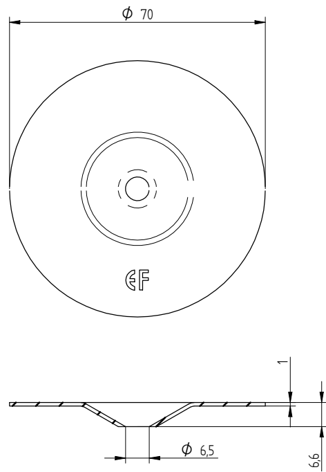
Eurofast DVP-EF-7010D
