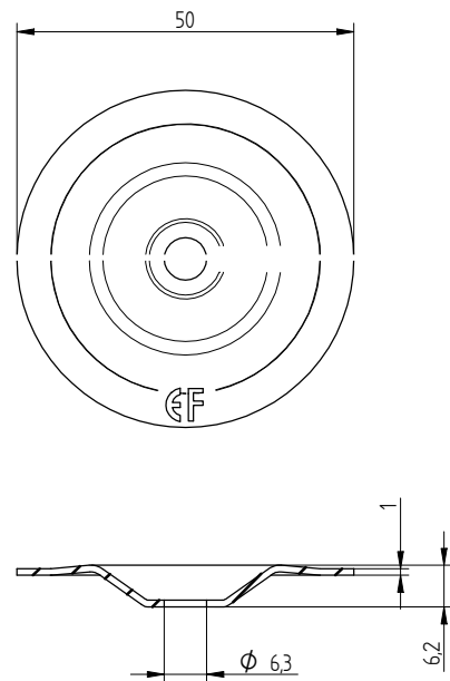
Eurofast DVP-EF-5010D
