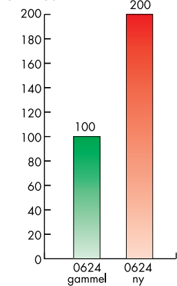
Sammenlikning av dreiemoment i % Bor Ø6mm boreddybde 18mm
