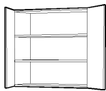
4012/4010 Høyde 704 mm Overskap 2 hyller 60, 70, 80, 90, 100 cm
