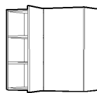
4021 Høyde 704 mm Hjørneoverskap med blindfelt 50 cm, 2 hyller 80 cm
