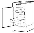
2441/2611 Høyde 704 mm Benkeskap, 1 skuff 2 lave innv.sk. 40, 50, 60 cm
