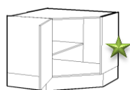
2082 Høyde 704 mm Hjørnebenk, dør i 45° 1 hylle 90 x 90 cm
