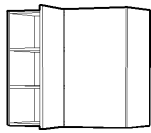
4020 Høyde 704 mm Hjørneoverskap med blindfelt 40 cm, 2 hyller 80 cm
