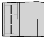
4420 Høyde 704 mm Hjørnevitrineskap blindfelt 40 cm, 2 glasshyller 80 cm
