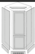
7073 Høyde 1952 mm Innbyggingsenhet for kjølehjørne 105 x 105 cm
