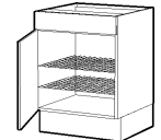
2104 Høyde 704 mm Benkeskap for int. av platetopp, 2 gryterister 60 cm
