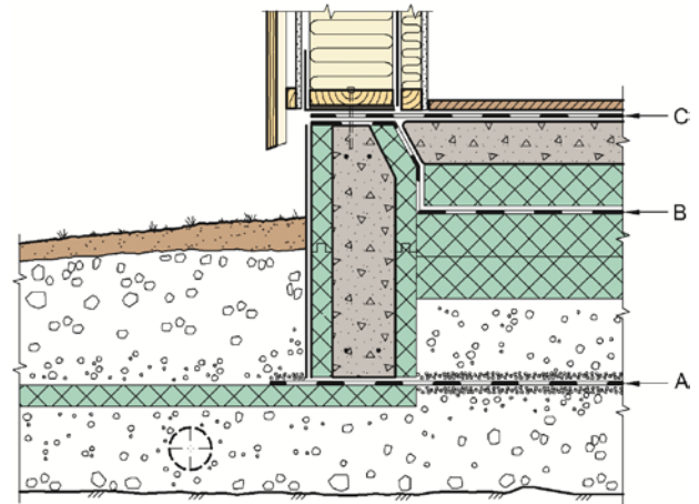
Fig. 1 Prinsipiell plassering av radonsperre i ulike bruksgrupper. Radonsystem Radonsperre er godkjent i bruksgruppe B.
