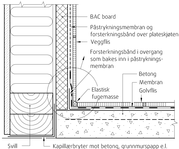
Fig. 3 Eksempel på overgang mellom flisledt golv og vegg med membran under flisene på golv.
