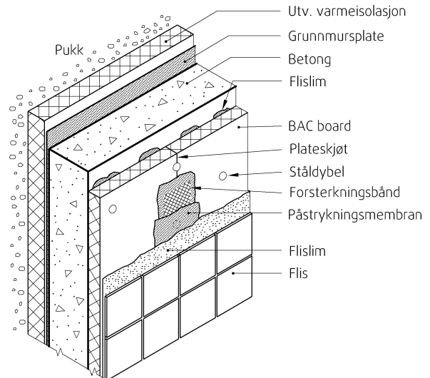
Fig. 4 Eksempel på bruk av BACboard på vegg under terreng.
