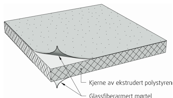
Fig. 1 Oppbygningen av BACboard. Platene er symmetriske med armert mørtel på begge sider.
