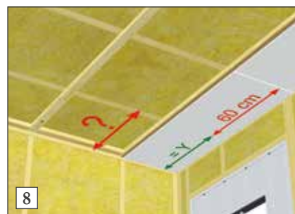
8) For å finne lengden på 1. plate i 2. platerad tar man lengden på 1. plate i 1. platerad minus 60 cm.
