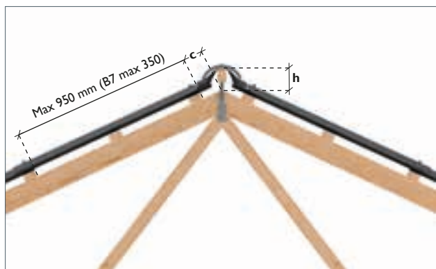
2 Cembril Konisk rygning med Cembril Rygningsbånd
