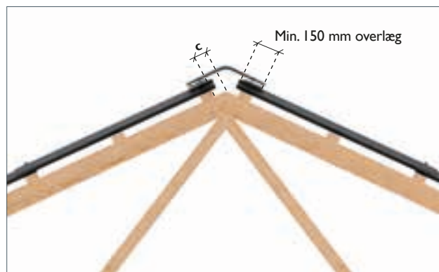
3 Cembril Vinkelrygning og Cembril Element til tagrumsventilation
