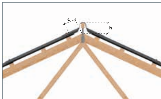
4 Cembril Todelt bølget rygning
