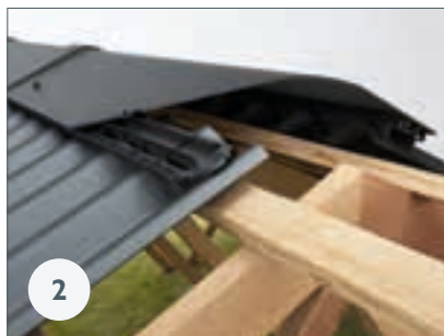
2 Ventilation ved rygningen kan etableres ved brug af Cembrit Rygningselement, se s. 16.
