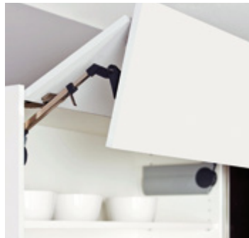
Skap med topphengslet foldedør. Praktisk f. eks. når man rydder ut av oppvaskmaskinen, døren er ikke i veien. Fåes til K-høye skap. Ikke til klassiske dører.
