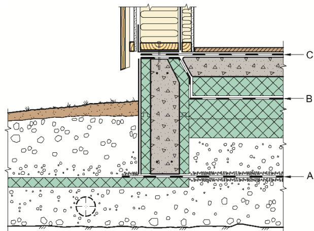
Fig. 1 Prinsipiell plassering av radonsperrer i ulike bruksgrupper. Canes Radonsperre er godkjent i bruksgruppe B.
