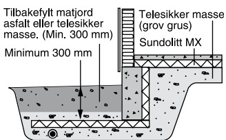
Ringmursfund. oppvarmet bygning
