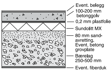
Prinsipp for oppbygging av industrigulv
