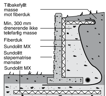
Prinsipp for isolering av støttemur
