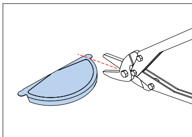
Klipp av eller brett "øret" som ikke blir brukt (det som vender inn mot taket).
