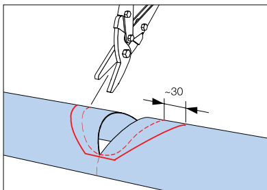
Lag hullet ferdig ved å klippe slik som vist på bildet.
