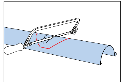
Bruk en baufil til å lage et hull i rennen.
