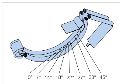
SSK takrennekroken kan justeres i forskjellige takvinkler.
