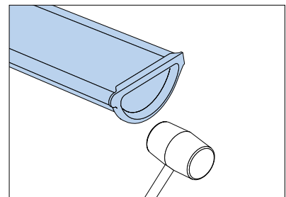
Endebunn RG er selvforsegkende og kan bli brukt både på venstre og høyre side av rennen. Bruk en gummihammer for å slå den på plass.
