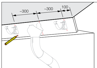
Marker SSK krokene rundt nedløpsrøret.
