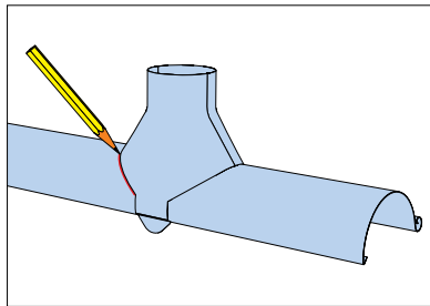
Bruk nedløpskummen som en mal på rennen.
