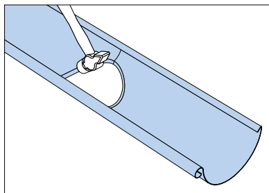
Bruk en hammer på kantene for å få et jevnt vannfall.
