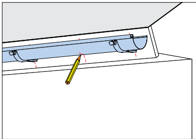
Plasser rennen i krokene og marker nedløpskum OMV på rennen.
