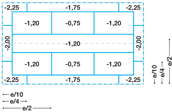
Takvinkel 20°
