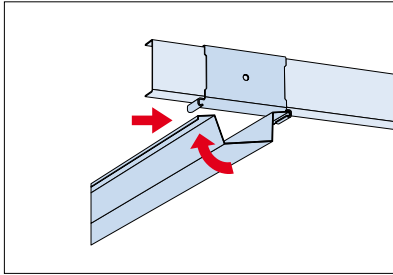
Fest sekundærprofilen (S) til beslaget (PS).
