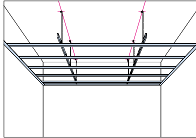
Sikre hver femte PS med en selvborende skrue.
