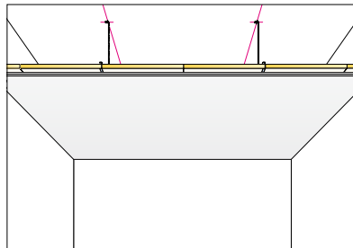
Monter plater i henhold til produsentens anvisning.
