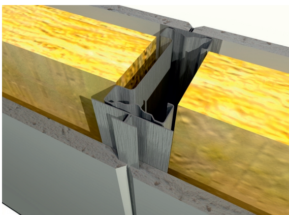
Uni Wall plateskjøt
