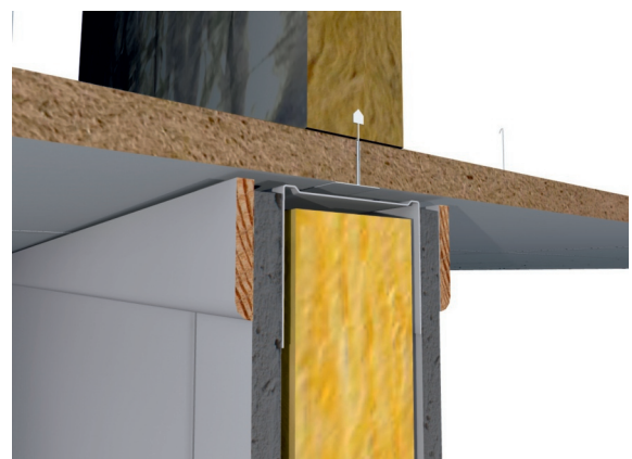
Uni Wall med trebelistning mot lydsperre
