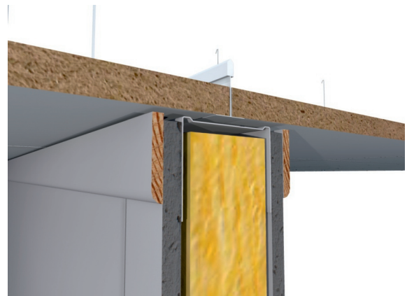
Uni Wall med trebelistning mot himling
