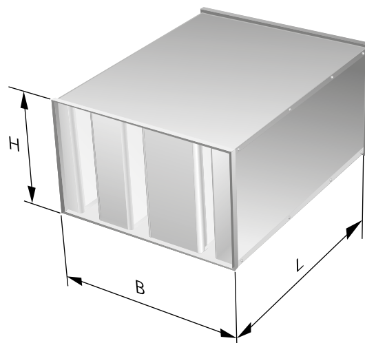
Figur 4. CADENZA, måttskiss
