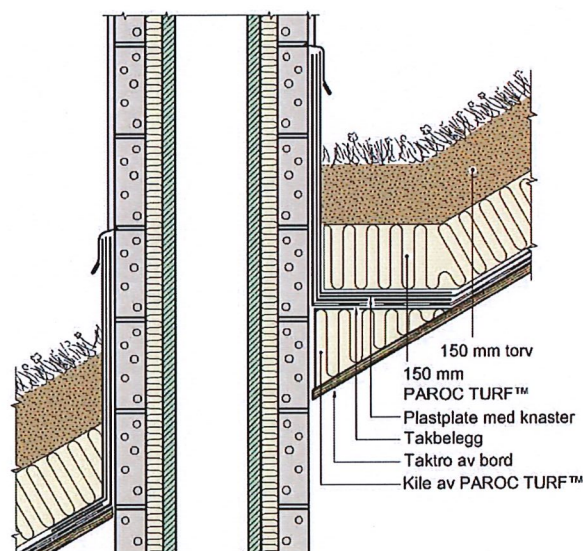
Fig. 4 Eksempel på gjennomføring av pipe.
