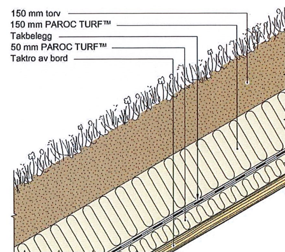
Fig. 5 Eksempel på PAROC TURF™ med tilleggsisolasjon under takbelegget.
