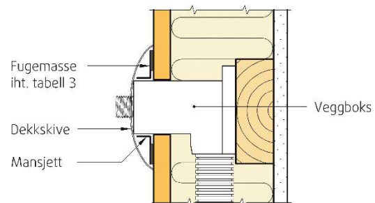
Fig. 3 Rørgjennomføring hvor mansjettene limes fast til baderomspanelet
