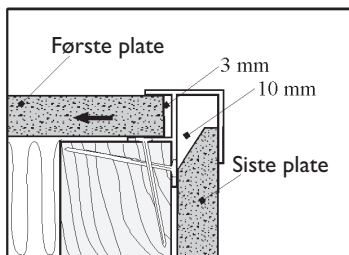
Fig. 5 Utvendig hjørne
