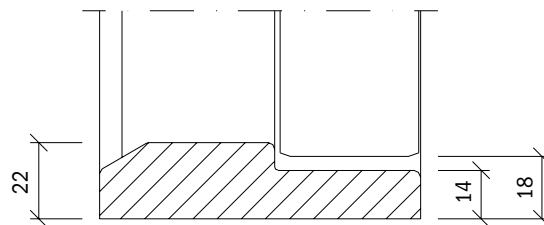
Standard terskel av eik Kode E
