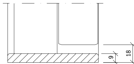
Terskelplate av eik, mellomliggende (9 mm spalte) Kode B
