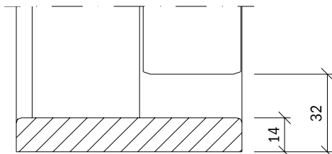
Flat underliggende terskel av eik. NB! Øker karmytterhøyden med 14 mm. Kode Z
