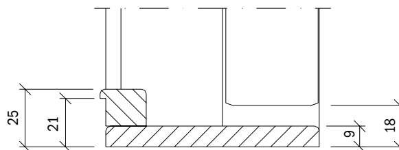
Terskelplate av eik med list for gulvbelegg, mellom-liggende (9 mm spalte). Kode BB
