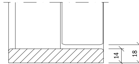
Flat mellomliggende terskel av eik. (4 mm spalte) Kode S
