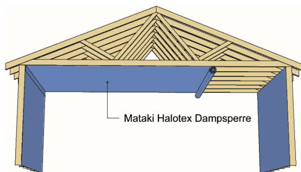
Fig. 2 Mataki Halotex Dampsperre montert i yttervegger og mot kaldt loftsrom
