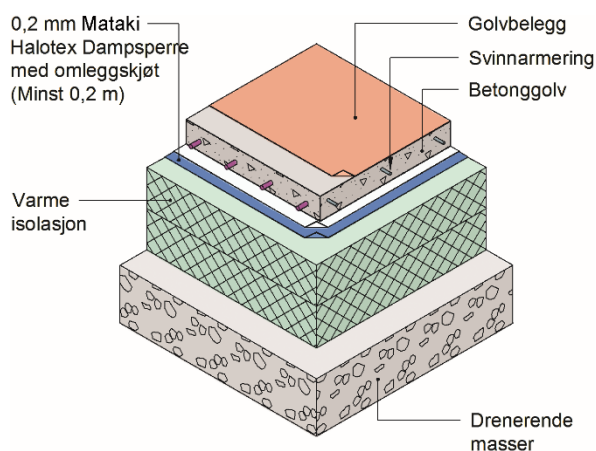
Fig 3 Mataki Halotex Dampsperre montert i betonggolv på grunnen
