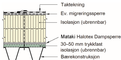
Fig. 1 Mataki Halotex Dampsperre montert i massiv takkonstruksjon
