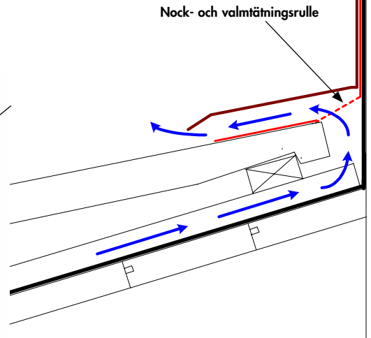
Bild 3: Väganslutning, montage dold avrinning höjdded. Sörj för god ventilation vid denna montering.
