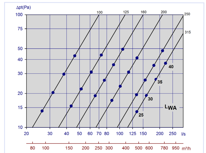
Diagram 46: TLG-G i kanal ende, tilluft
