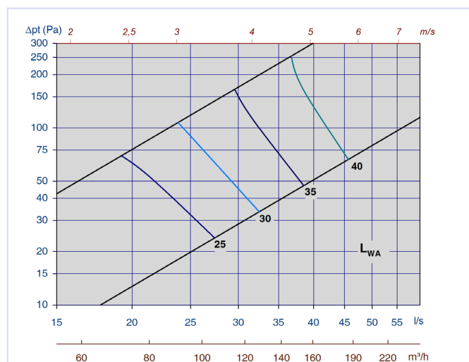
Diagram 4: TLG-G m/Luna 100-125 min. spalt, tilluft
