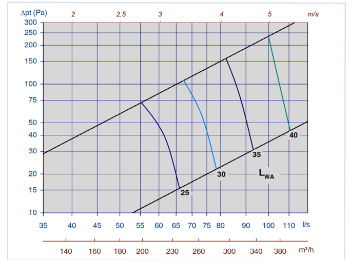
Diagram 42: TLG-G m/Luna 250-315 maks. spalt, tilluft
