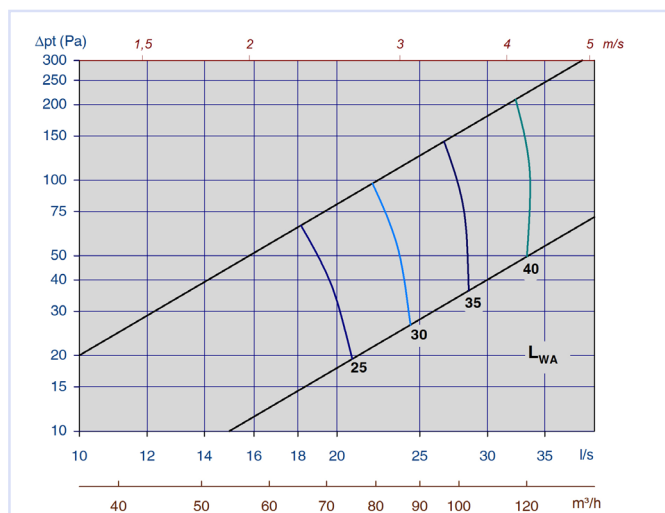
Diagram 2: TLG-G m/Luna 100-100 midt. spalt, tilluft
