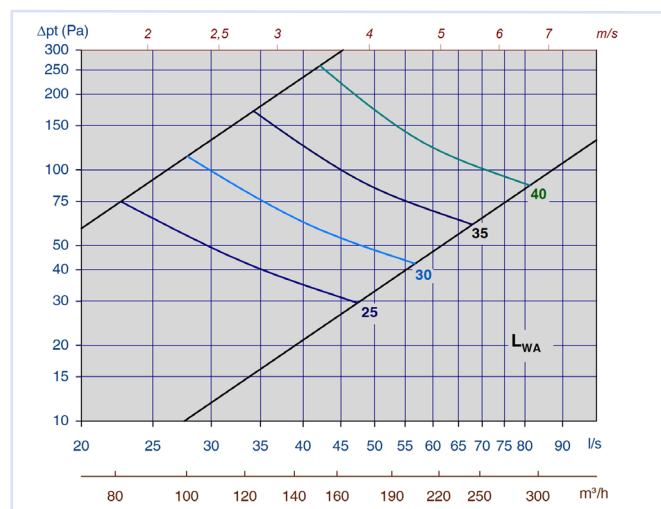
Diagram 54, TLG-G m/Luna 125-160, midt spalt, avtrekk
