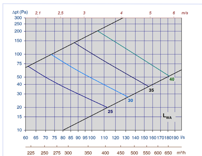
Diagram 69, TLG-G m/Luna 200-315, midt spalt, avtrekk
