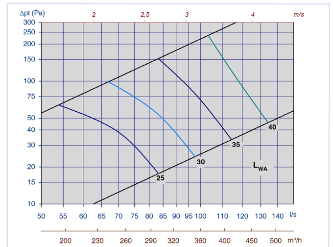
Diagram 44: TLG-G m/Luna 315-315 midt. spalt, tilluft
