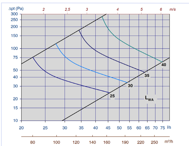
Diagram 15: TLG-G m/Luna 125-160 maks. spalt, tilluft
