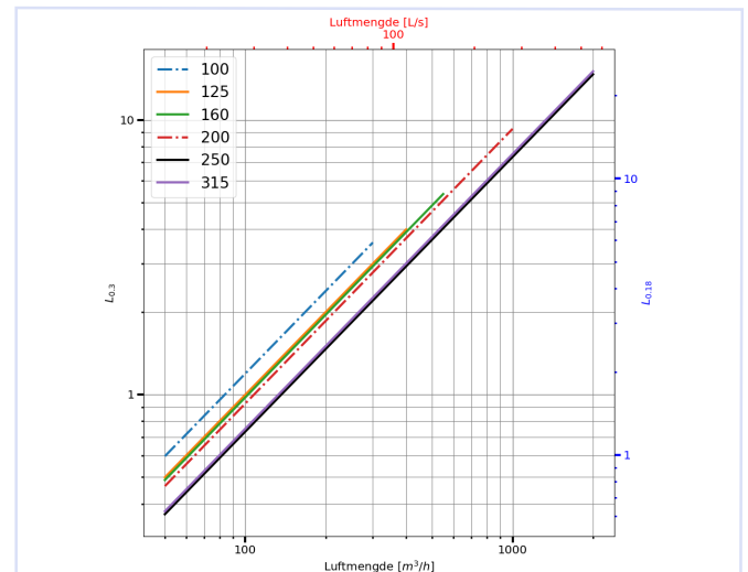
Diagram 83, kastelengde sluttastighet 0,3 og 0,18 m/s.
