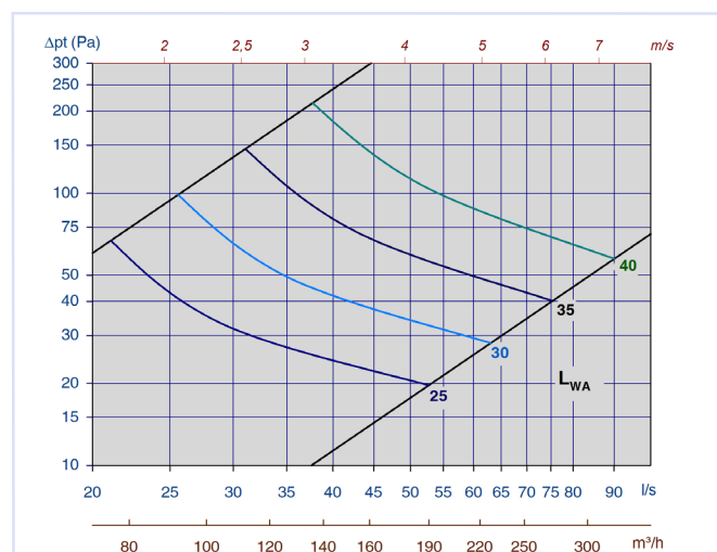
Diagram 58, TLG-G m/Luna 125-200, maks spalt, avtrekk
