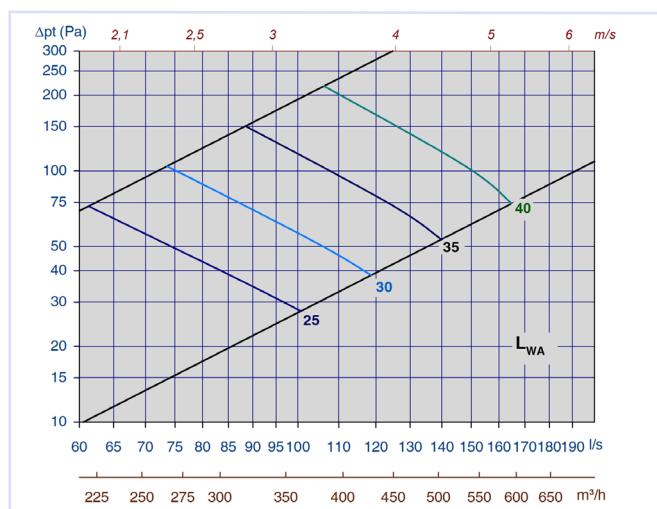
Diagram 66, TLG-G m/Luna 200-250, midt spalt, avtrekk
