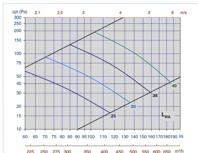
Diagram 70, TLG-G m/Luna 200-315, maks spalt, avtrekk
