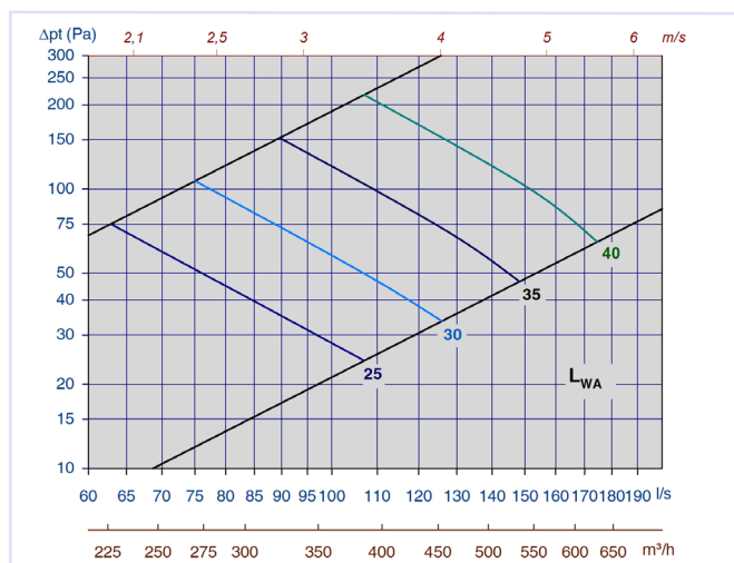
Diagram 67, TLG-G m/Luna 200-250, maks spalt, avtrekk
