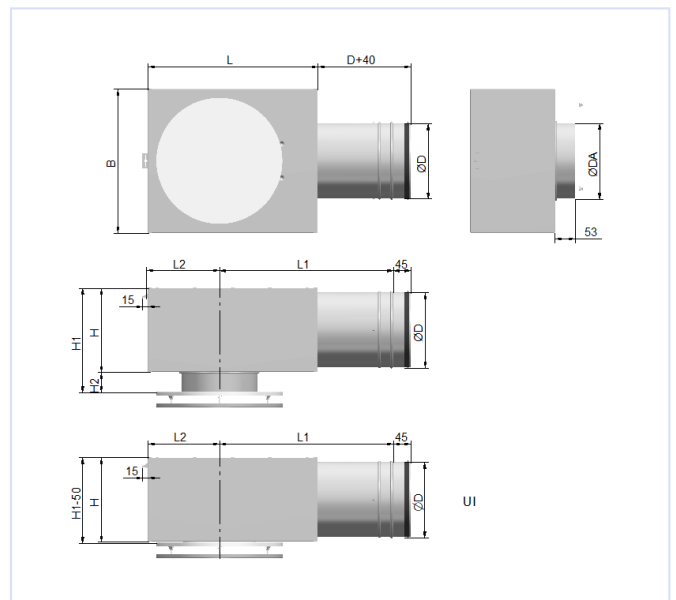
Figur 2, målskisse TLG-G med Luna
