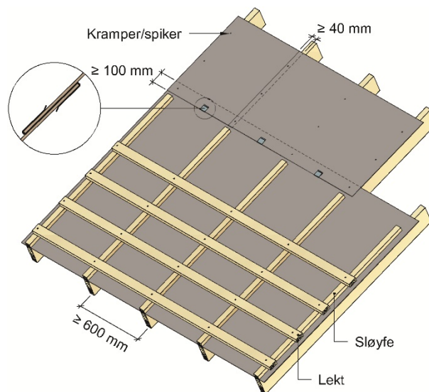
Fig. 1 Hunton Sutak legges i forband. Bruk av klips i plateskjøtene forenkler monteringen og reduserer faren for inndrev av regn- og snø.
