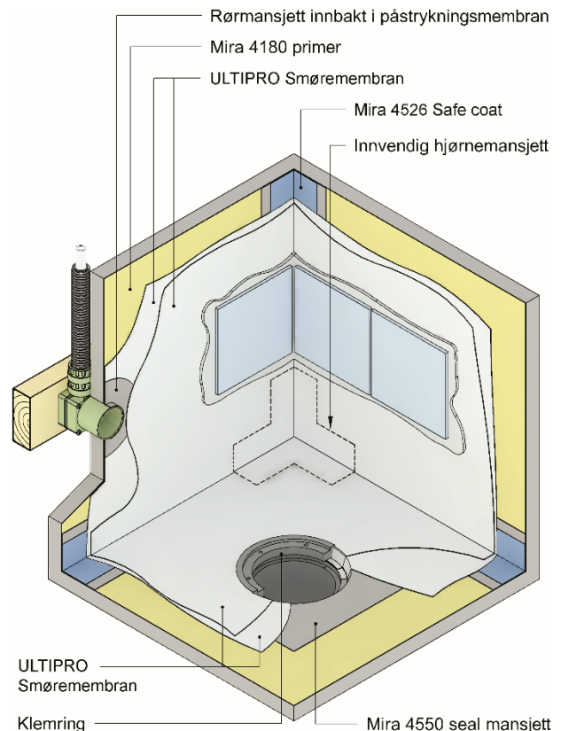
Figur 1 Oppbygging av ULTIPRO Smøremembransystem
