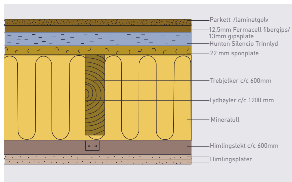
Figur 1 Anbefalt oppbygning av gulv med parkett på Silencio Thermo på trebjelkelag med lydhimling av to-lags lydstrålingsminskende kledning (f.eks. 12,5mm Fermacell fibergips med rett kant/13mm gips/12mm spon/11mm trefiberplater for vegg/himling).
